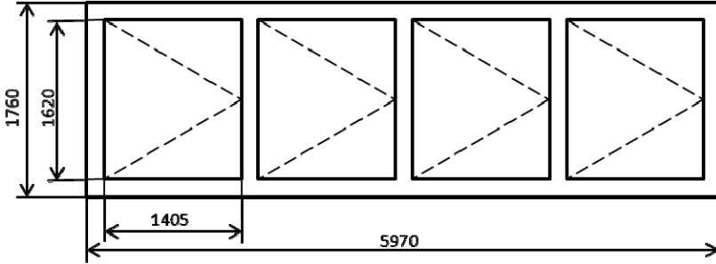
Рис. 2. Схема оконного переплета
