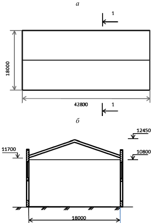
Рис. 1. Производственное здание: a – план; b – разрез (1–1 на рис. 1 a ). Размеры указаны в мм
