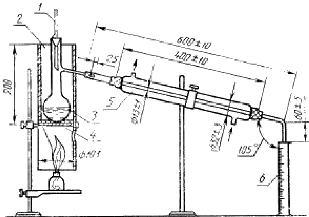
1—термометр; 2, 4—металлические кожухи; 3—колба, 5—холодильник; 6—цилиндр
